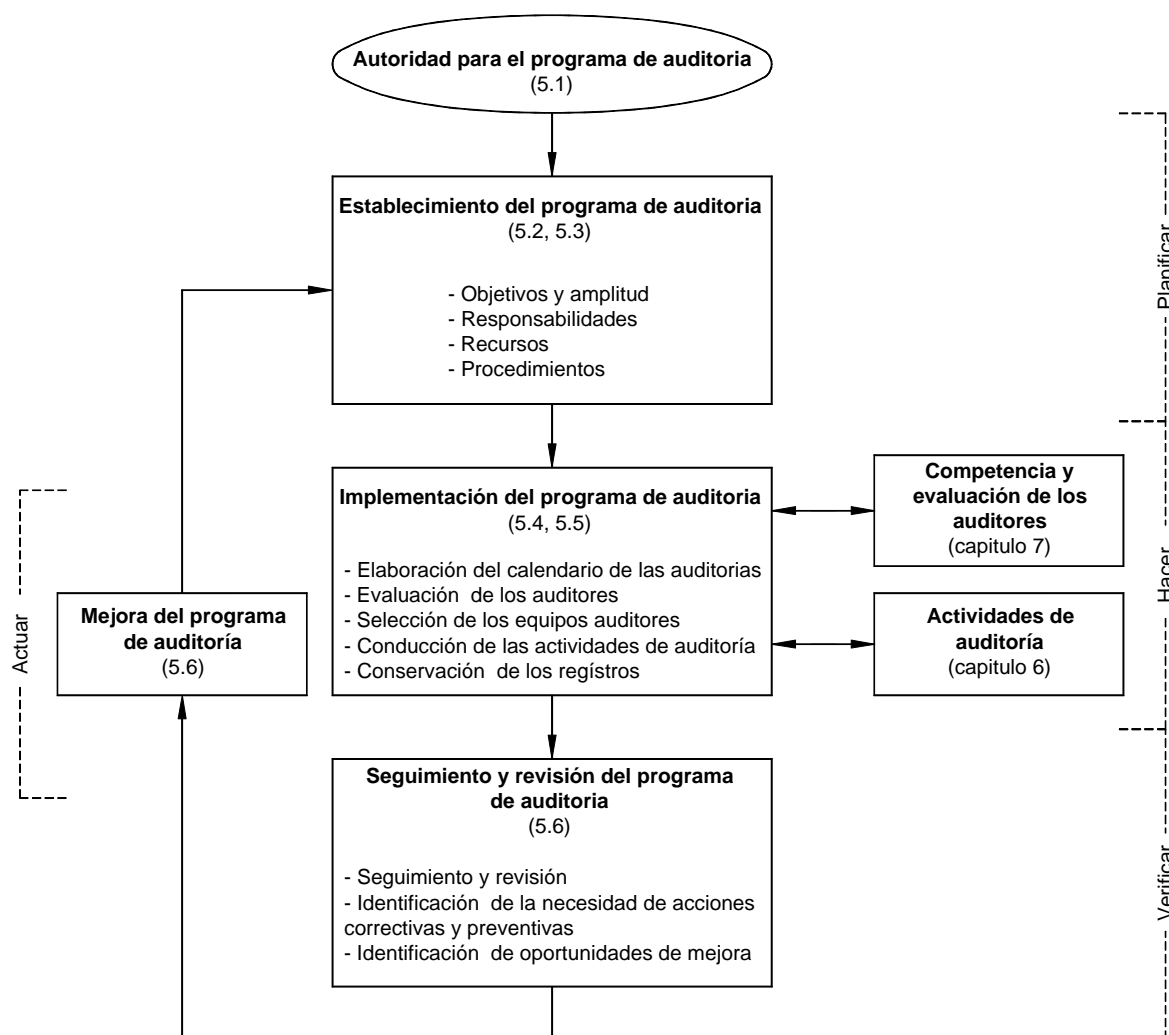
Figura 1. Diagrama de flujo del proceso para la gestión de un programa de auditoría
